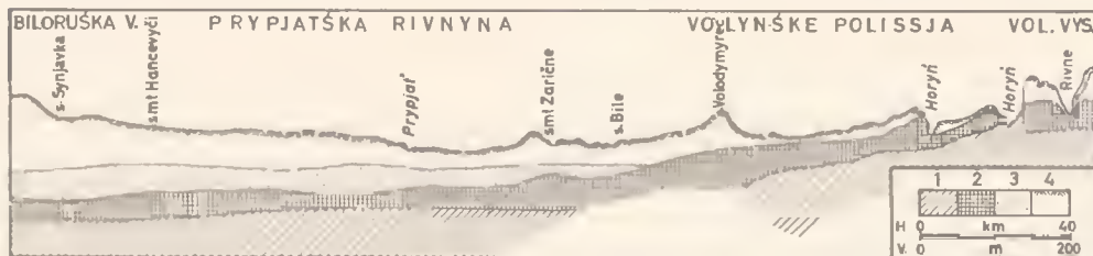
Схематичний геологічний профіль Полісся 1 — докембрій і палеозоікум. 2 — Крейда. 3 — Палеоген. 4 — Сучасний ґрунт. Vys. — Височина. Vol. vys. — Волинська височина
